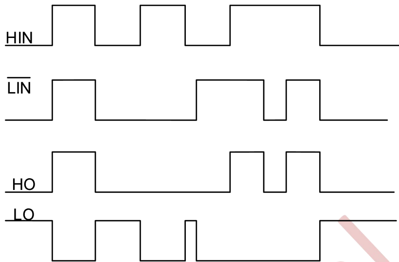
图 9-1 G2020Q 输入输出时序波形
